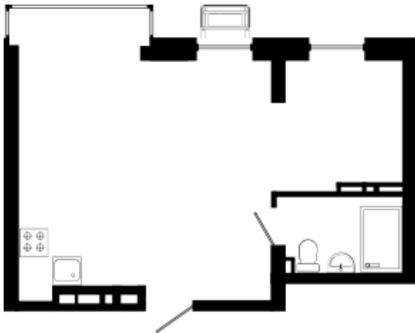
Планировка квартиры
